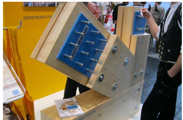
Verbindungsdetail im Hallenbau
